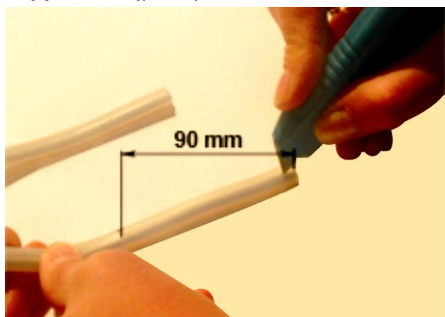
1. Разрезать изоляцию(90мм)
