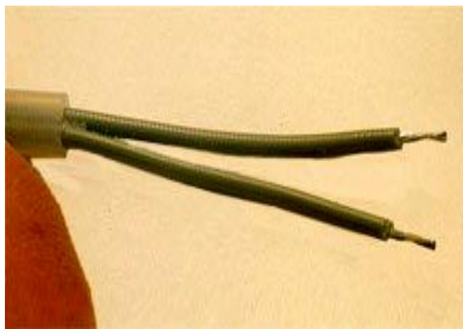
5. Разделить контакты
