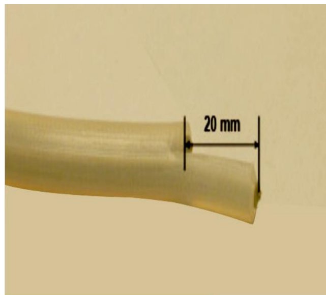
2. Отрезать нагревающий элемент на 20 мм Срез изолировать силиконовой резиной
