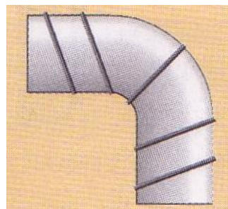
Регулярный шаг, соседние витки не должны соприкасаться на внутренней стороне
